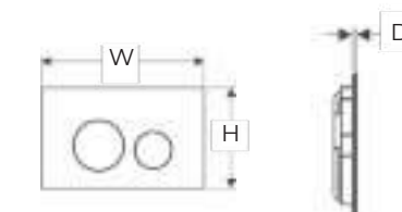
246 (W) x 152 (H) x 4 (D) mm
