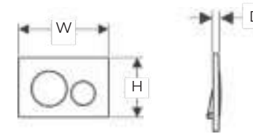
246 (W) x 164 (H) x 12 (D) mm
