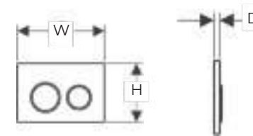
212 (W) x 142 (H) x 10 (D) mm
