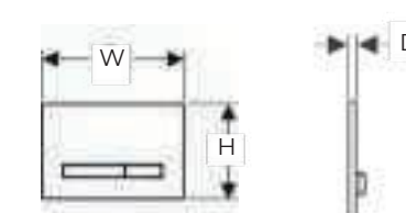
246 (W) x 164 (H) x 10-14 (D) mm
