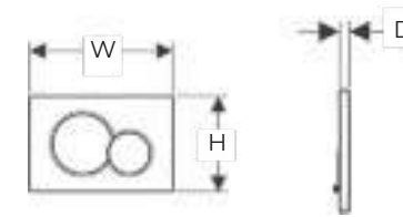
246 (W) x 164 (H) x 13 (D) mm
