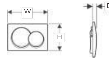
213 (W) x 142 (H) x 16 (D) mm
