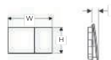
250 (W) x 146 (H) x 23-25 (D) mm
